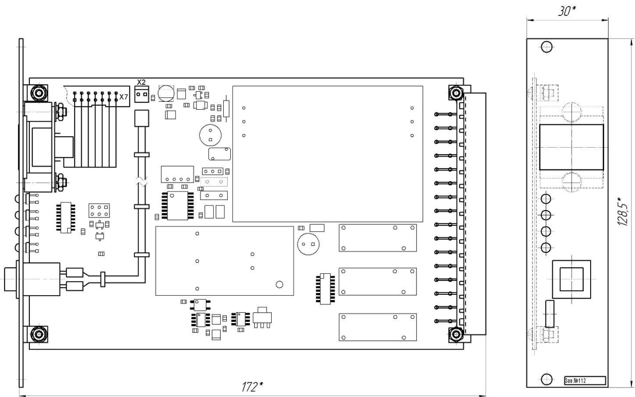
Рисунок Д.1 – МВП. Габаритные размеры
